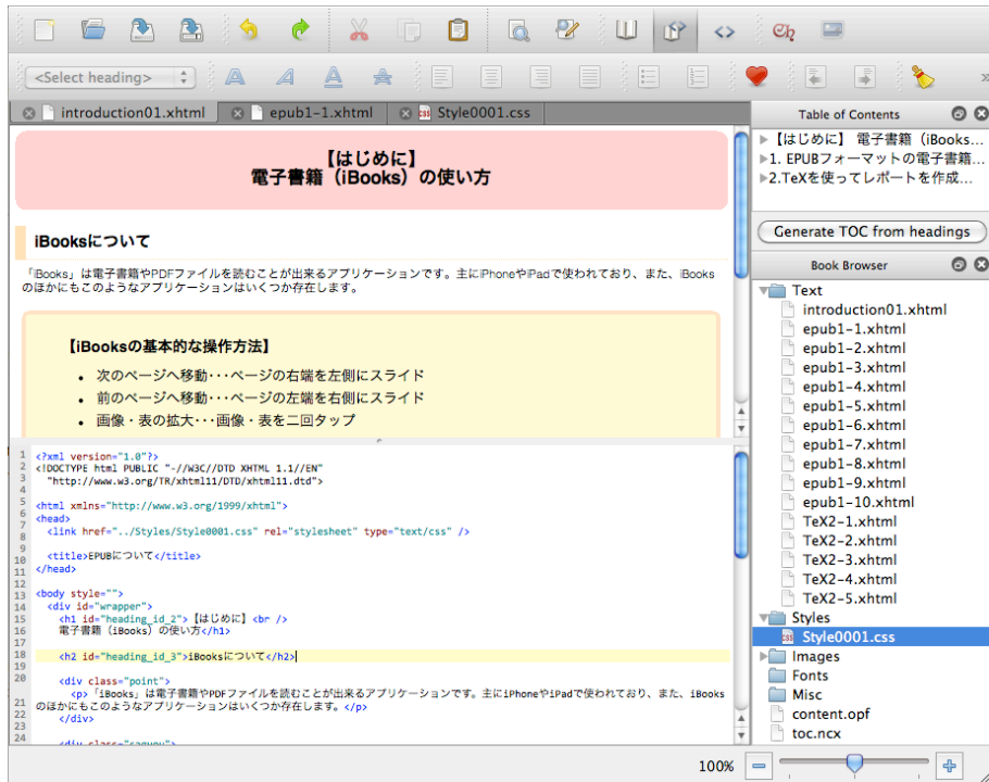
図 3 Split View
