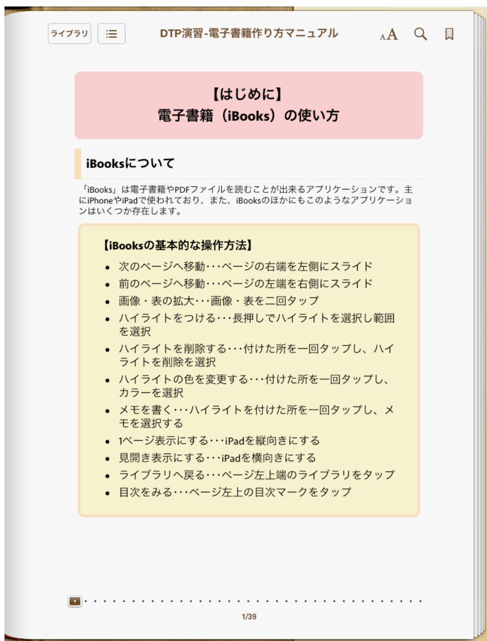
図4 はじめに
