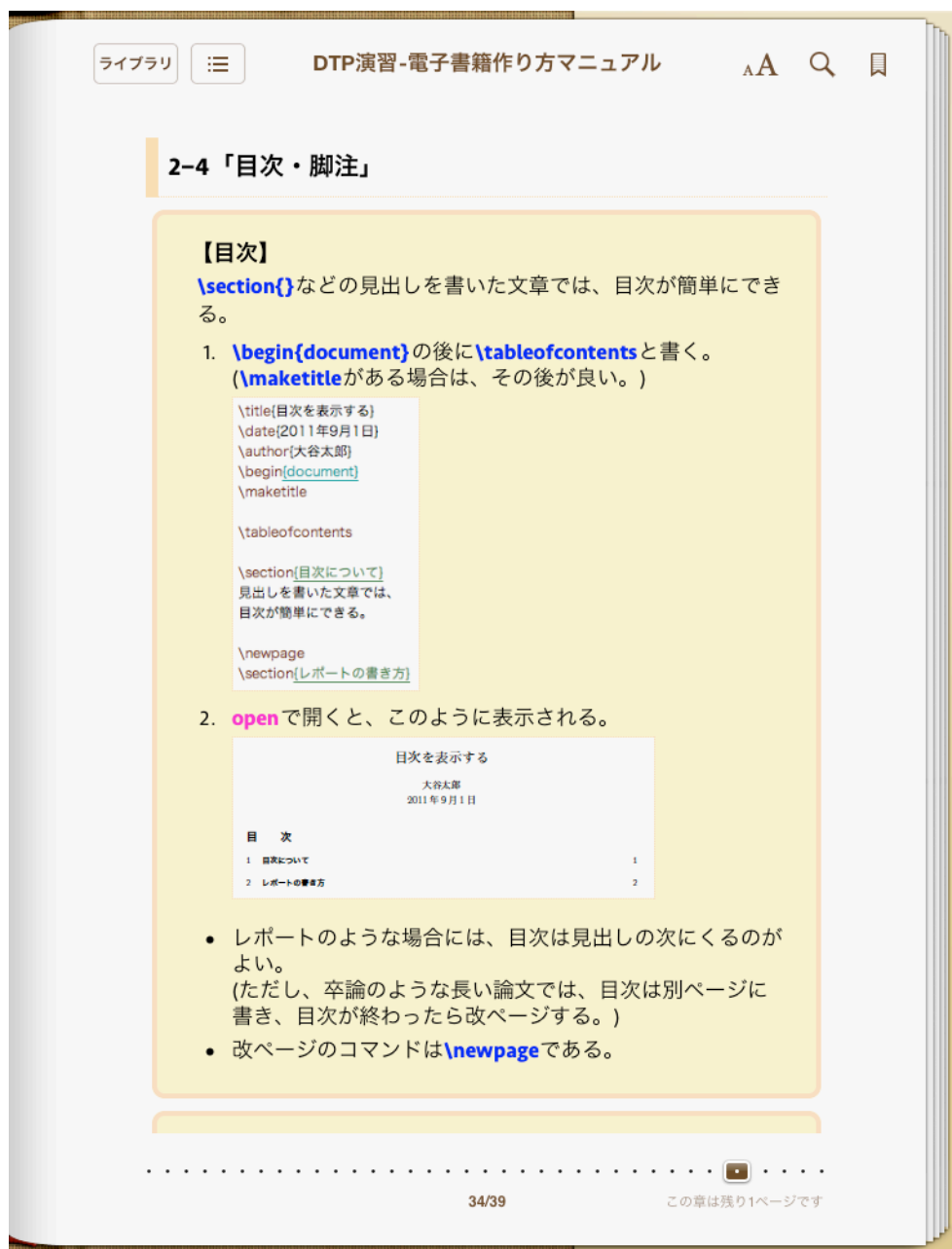
図 1 9 2-4 「目次・脚注」
