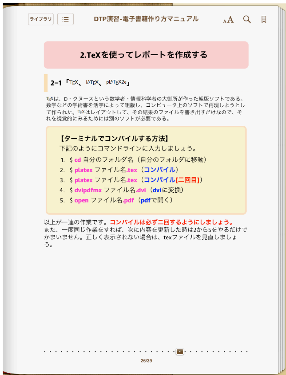
図 1 6 2-1 「TeX、LaTeX、pLaTeX2e」
