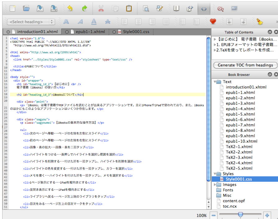
図 2 Code View
