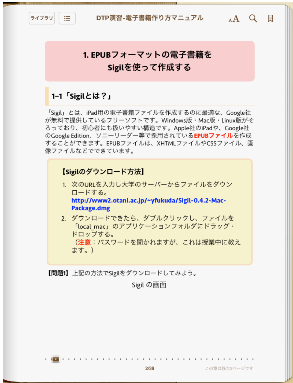
図 5 1-1 「Sigil とは？」
