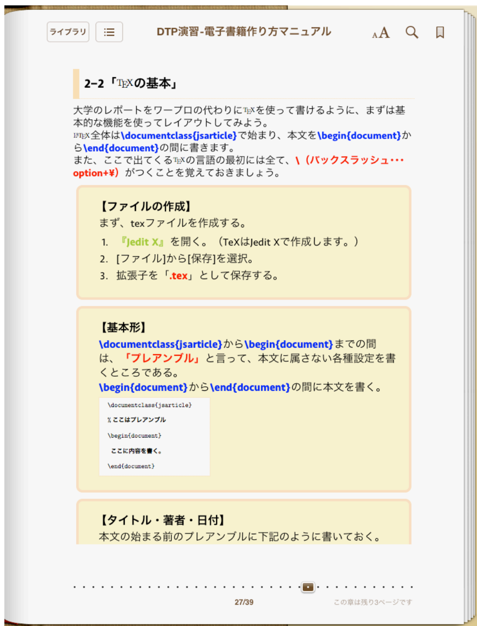
図 1 7 2-2 「TeX の基本」
