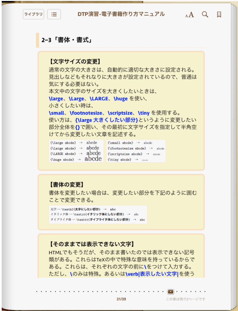
図 1 8 2-3 「書体・書式」
