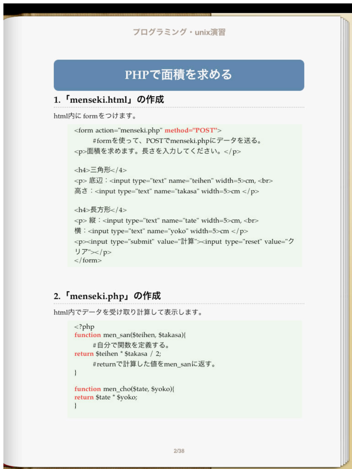
図 2 : PHP で面積を求める
